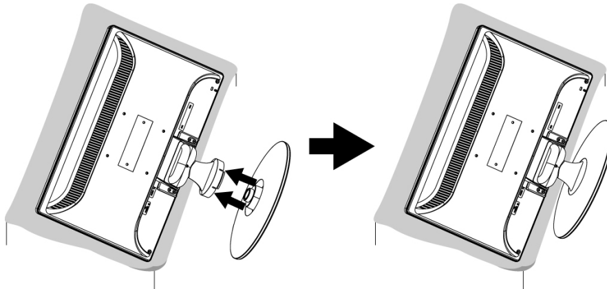
Bildschirmfuß montieren (Abb. ähnlich)
