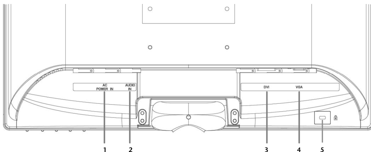
(Afb.: Aansluitingen op de achterkant)
