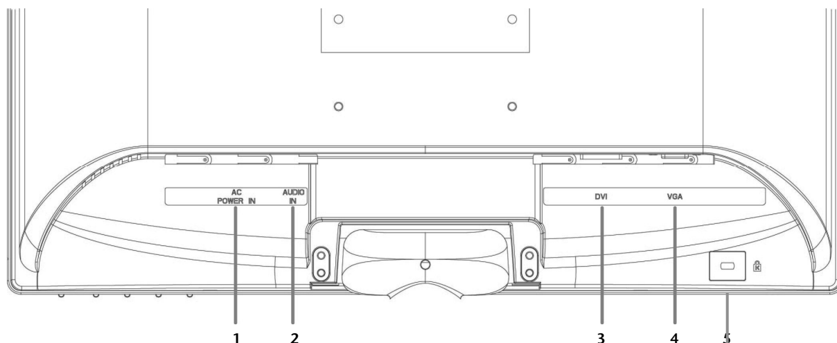
(III.: Tilslutninger bagside)
